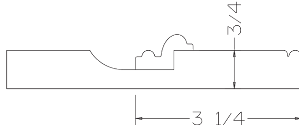
DOOR CROSS SECTION
